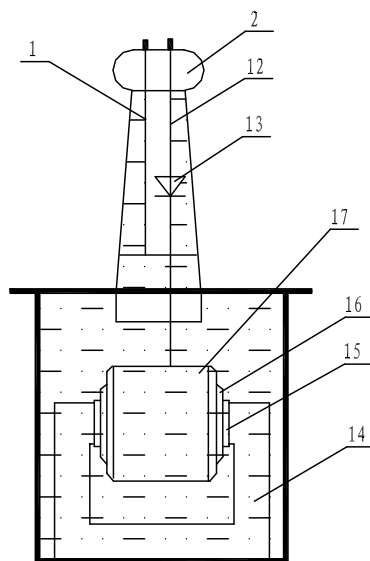
图 2：单台油浸式试验变压器内部结构图
