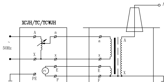
图 3：单台 YDJ 油浸式试验变压器原理图
